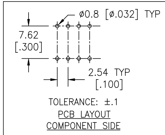
SRPG202SA SHOWN
